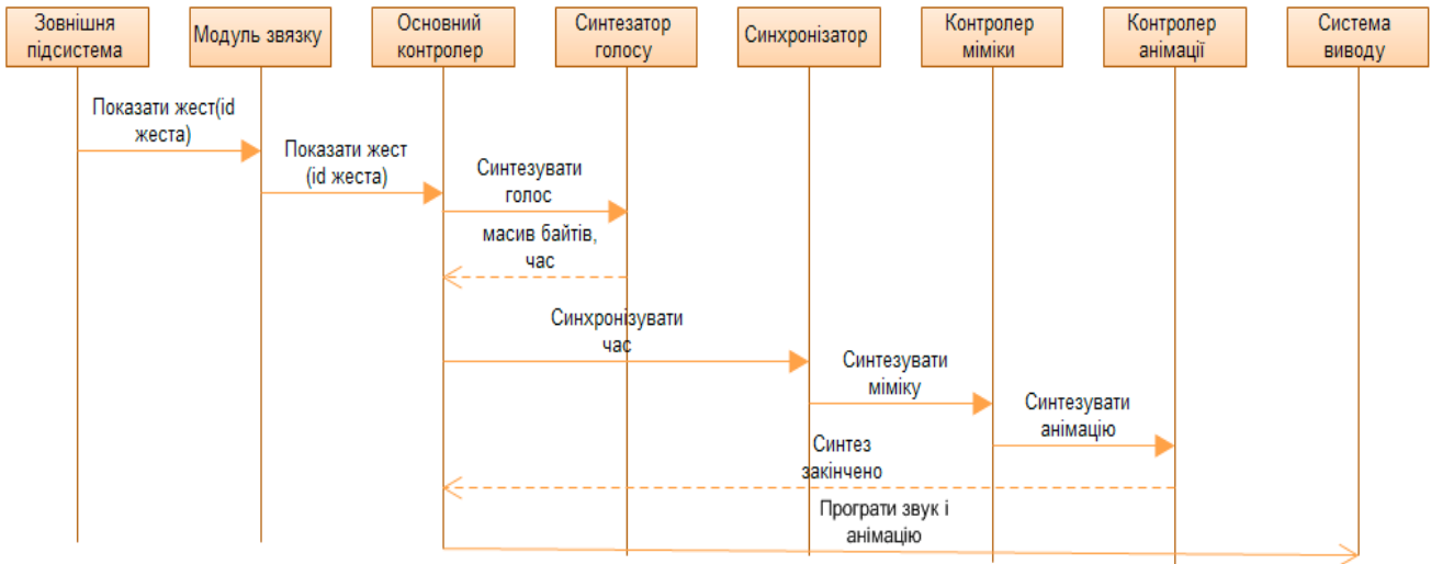
Рис. 5. Діаграма послідовностей
