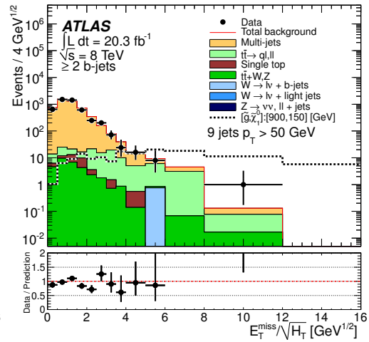
(f) 9j50, \geq 2 b -jets
