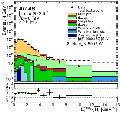
(e) 8j50, \geq 2 b -jets
