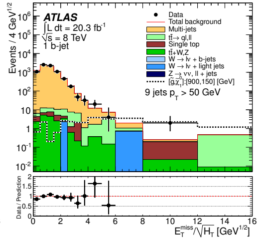
(d) 9j50, exactly one b -jet
