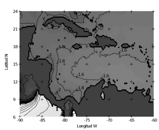
Figura 7. Fase anual en meses.
