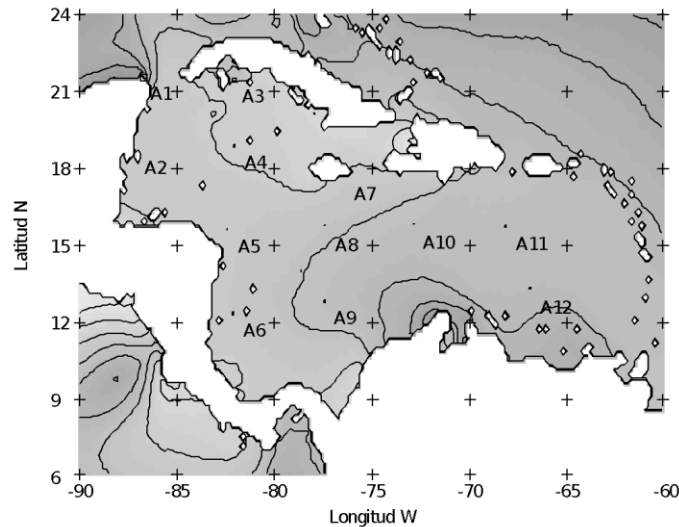
Figura 4. 12 Puntos dentro del MC seleccionados como representativos de la zona.
