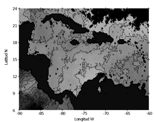
Figura 11. Fase trianual en meses.
