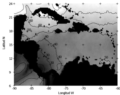
Figura 14. Varianza explicada anual [%].
