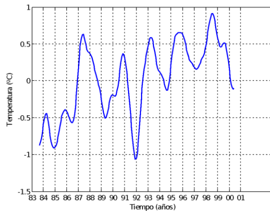
Figura 24. Serie filtrada a 6 meses en el punto A11.
