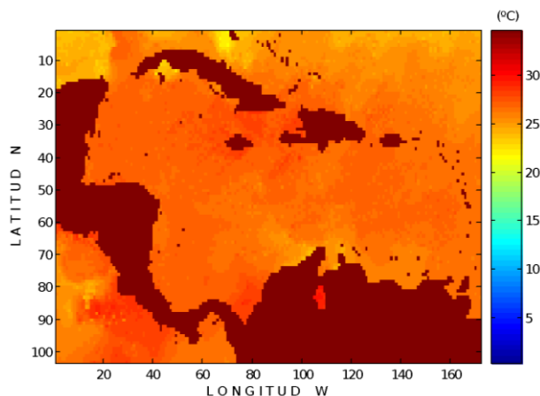
Figura 3. Imagen del día 4 de enero de 1984, que presenta información confiable. La temperatura se muestra por arriba de la media (~24 °C) con valores desde los 25°C hasta los 30°C. Los índices externos al MC fueron utilizados en la búsqueda de explicaciones de las anomalías de la TSM observadas. Estos índices son el Southern Oscillation Index (SOI) , Southern Oscillation Index extratropical (SOI*) , Northern Oscillation Index extratropical (NOI) , North Atlantic Oscillation Index (NAO) , Multivariate ENSO Index (MEI) ; y el North Pacific Oscillation (NPO) , oscilación
