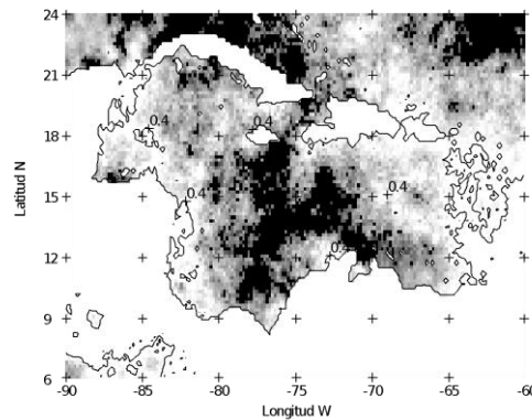
Figura 17. Varianza explicada cuatrianual. [%]
