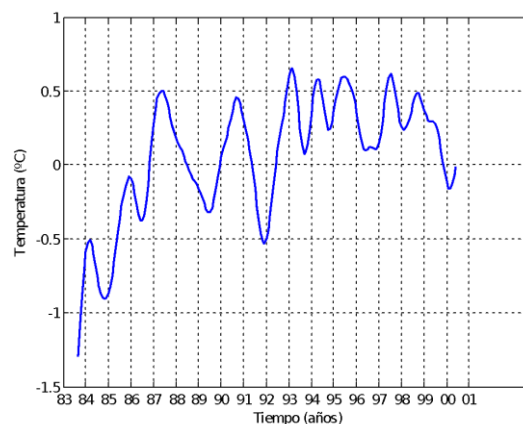
Figura 22. Serie filtrada a 6 meses en el punto A1.
