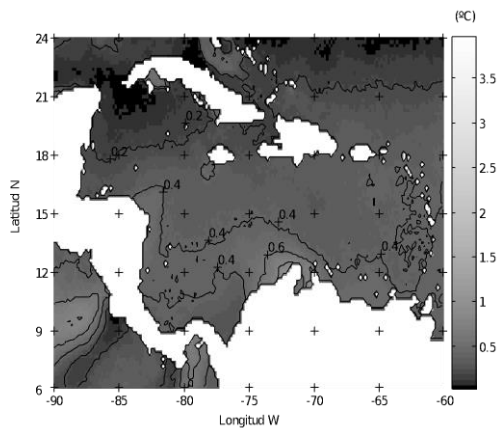
Figura 8. Amplitud semianual en °C.
