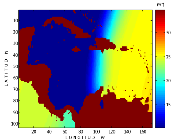
Figura 2. Imagen del día 29 de junio de 1982, que presenta información poco confiable. Se observa que los valores de temperatura para el MC son muy inferiores al promedio (24°C), con un mínimo de hasta 10°C.
