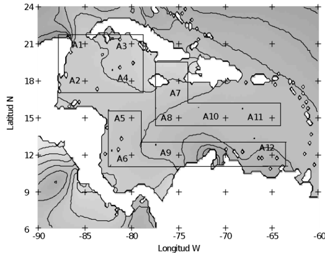
Figura 18. Regionalización del MC. Las regiones elegidas son los puntos A1, A2, A3 y A4, forman la región I; los puntos A5, A6, A9; y A12 la región II, y finalmente los puntos A7, A8, A10 y A11 la región III.
