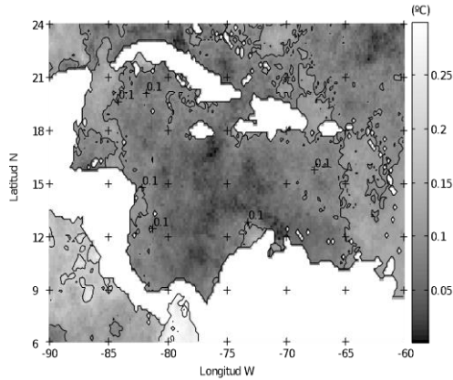
Figura 12. Amplitud cuatrianual en °C.
