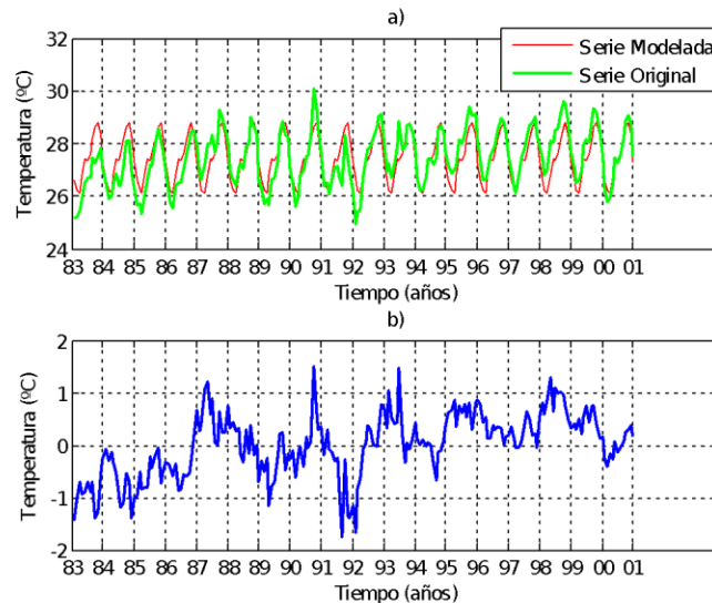
Figura 21. a) Serie modelada y serie original, b) anomalías en el punto A11, ( 15^{\circ}\text{N} , 65^{\circ}\text{W} ).
