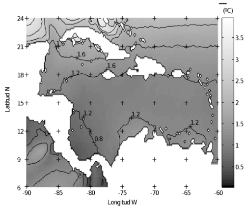
Figura 6. Amplitud anual en °C.
