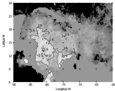
Figura 16. Varianza explicada trianual [%]
