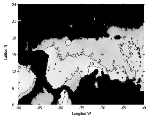
Figura 15. Varianza explicada semianual [%].
