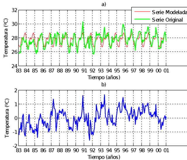
Figura 20. a) Serie modelada y serie original, b) anomalías en el punto A6, ( 12^{\circ}\text{N} , 80^{\circ}\text{W} ).
