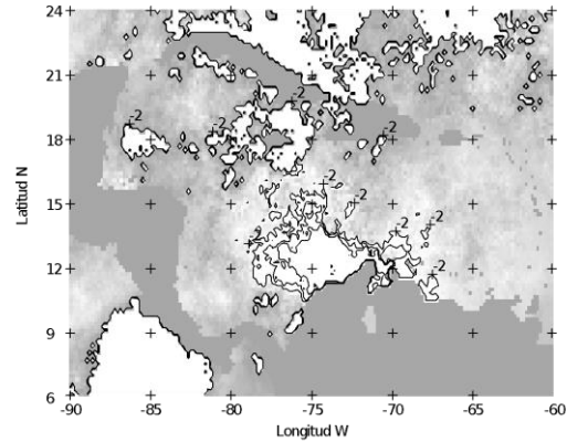
Figura 13. Fase cuatrianual en meses.
