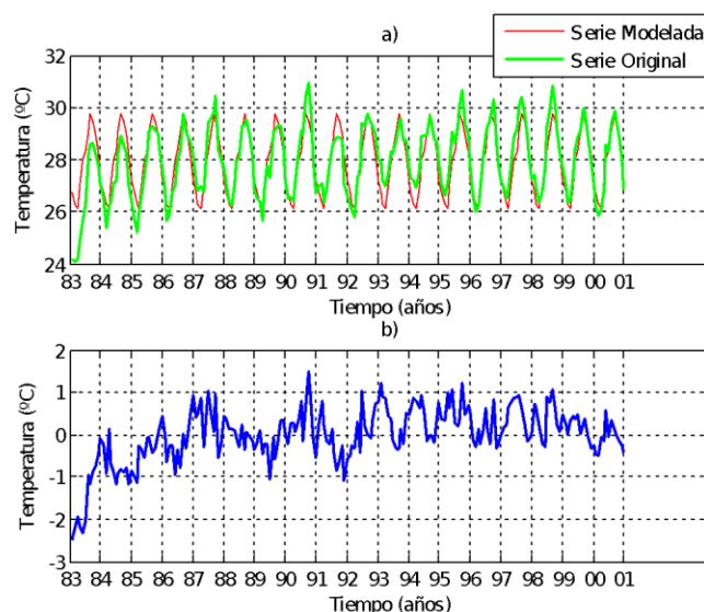
Figura 19. a) Serie modelada y serie original y b) anomalías en el punto A1, (21° N, 85° W).
