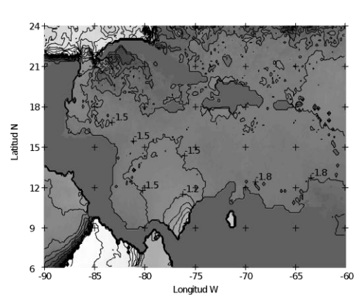
Figura 9. Fase semianual en meses.
