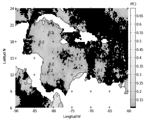
Figura 10. Amplitud trianual en °C.
