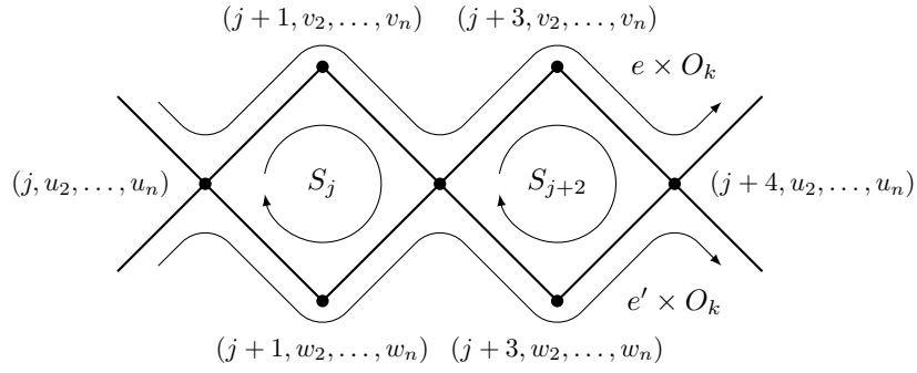
Fig. 4. Proof of Lemma V.6(2).
