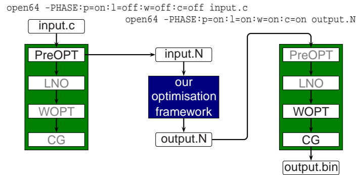
Fig. 27. Optimisation process
