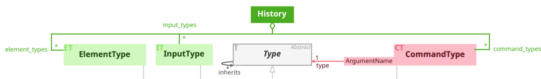
FIGURE 3.1 – Diagramme de classe des Types enregistrés dans l'historique. Les structures relatives aux données manipulées sont en vert, et celles représentant les changements effectués sont en rouge.
