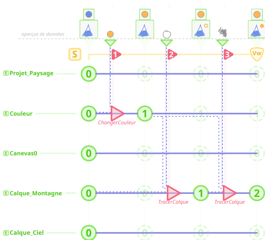
FIGURE 2.10 – Exemple de déroulement d’une Session d’édition. Les Elements utilisés dans cet exemple sont représentés à gauche. Des Commands ont été exécutées séquentiellement au cour d’une Session, générant des Changes représentés et numérotés sur la ligne de la Session. Ces Changes sont liés aux CommandVersions qui les composent. Les ElementVersions de chaque Element sont représentées sur une ligne par Element dans la frise, et liées aux CommandVersions les ayant générées. Les liens de parenté n’y sont pas représenté. Projet_Paysage est à la racine de la View, et possède Canevas0 et Couleur comme enfants. Canevas0 à son tour possède Calque_Montagne et Calque_Ciel comme enfants. Les états de Couleur et de Canevas0 sont illustrés en haut de la frise pour une meilleure visualisation. Le TRIP est représenté par les liens bleus entre Versions et la CommandVersion de la Command les ayant utilisées.
