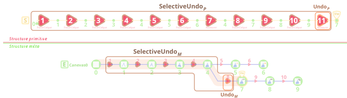
FIGURE 2.15 – Commands concernées par \text{Undo}_p et \text{Undo}_M .
