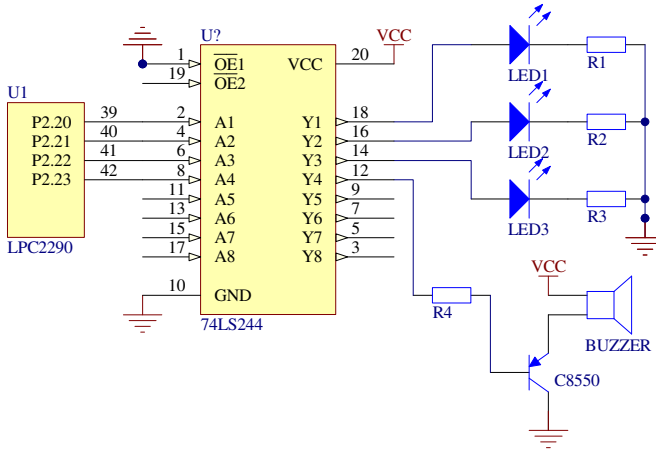
Fig. 3. Alarm Module
